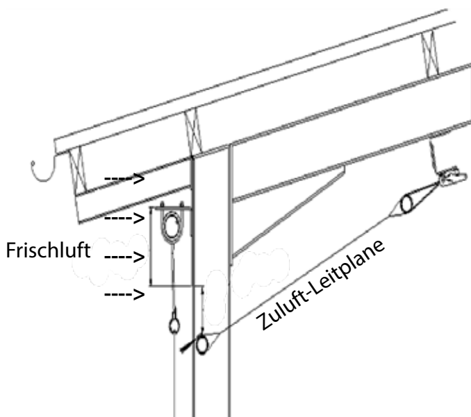
Schnittzeichnung der AGROTEL Zuluft-Leitplane
